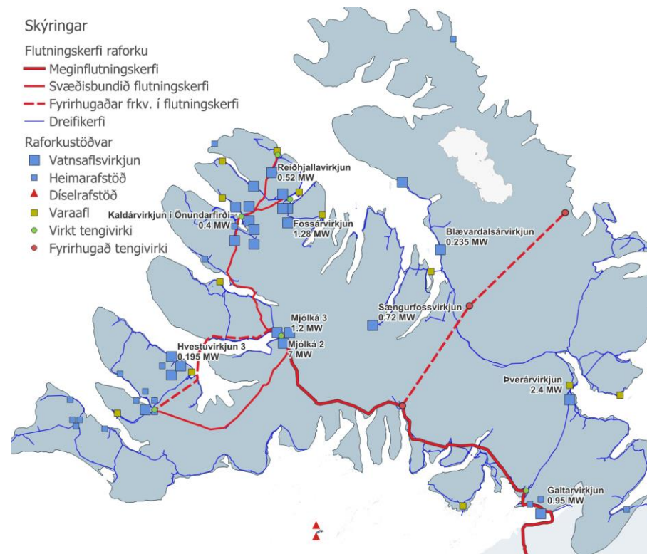
Mynd 4-10 Raforkuframleiðsla, flutningskerfi og dreifikerfi raforku.
