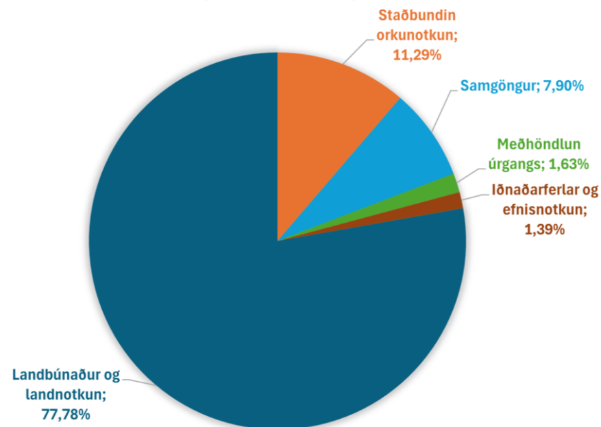
UPPSPRETTUR LOSUNAR GRÓÐURHÚSALOFTTEGUNDA Á VESTFJÖRÐUM (TONN CO2 ÍG)
