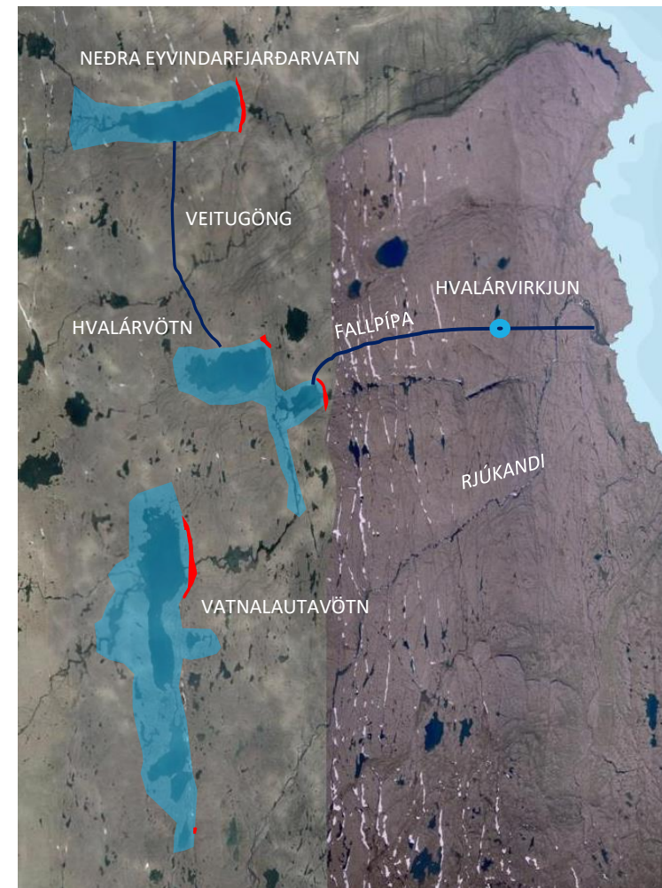
Mynd 3: Hvalárvirkjun ásamt uppistöðulónum
